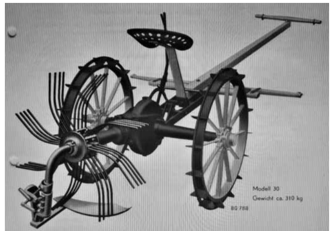
Kartoffelgraber Bucher-Guyer Mod. 30, Gewicht 310 Kg, Bucher-Guyer Maschinenfabrik, Niederweningen ZH (Foto aus Internet)
